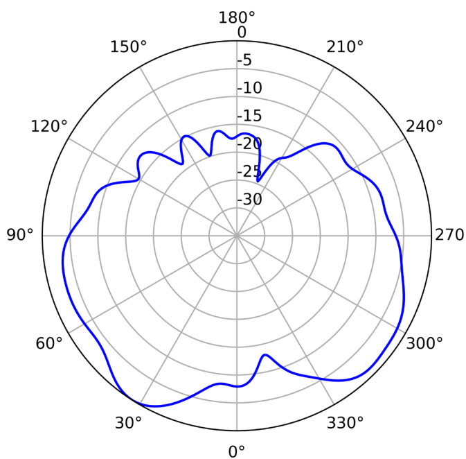
5GHz (Vertical)
